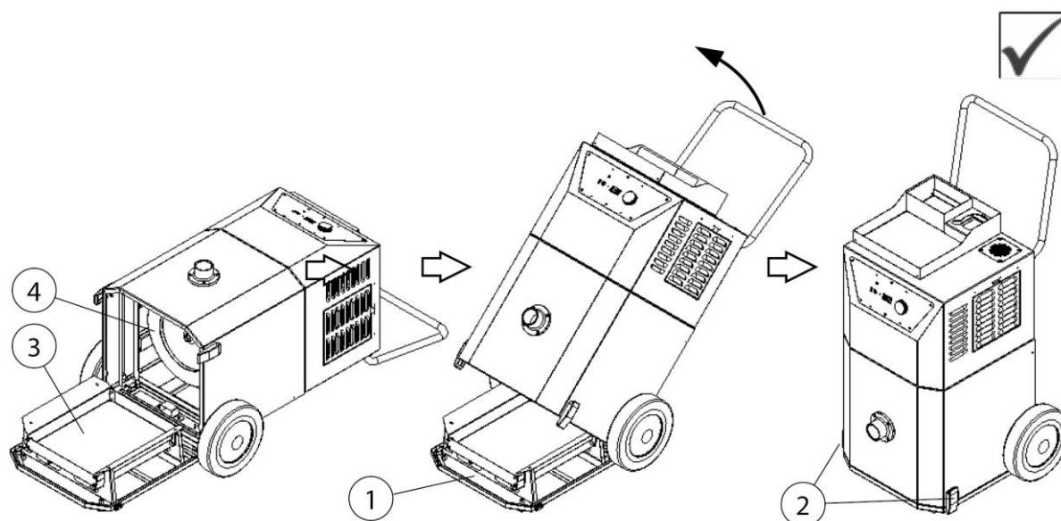
Rys. 13: Zamykanie pokrywy serwisowej
