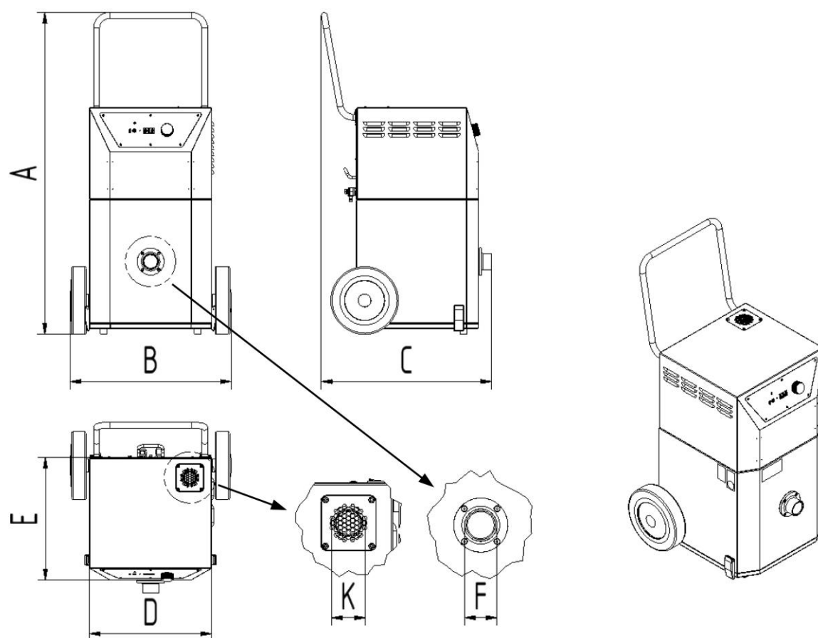
Rys. 15: Karta wymiarów
