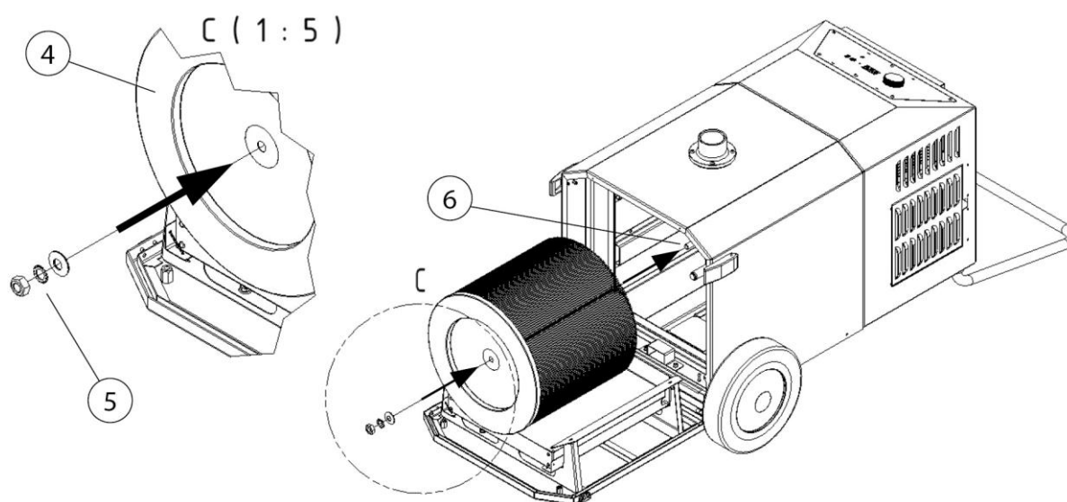
Rys. 12: Włożyć nowy wkład nabojewy
